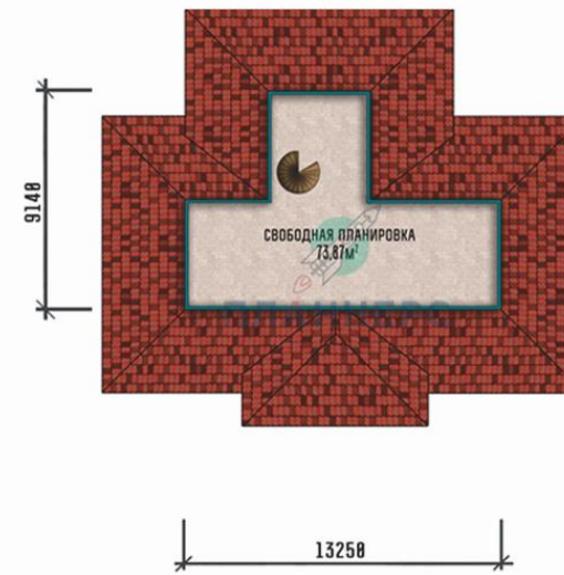
План мансардного этажа
