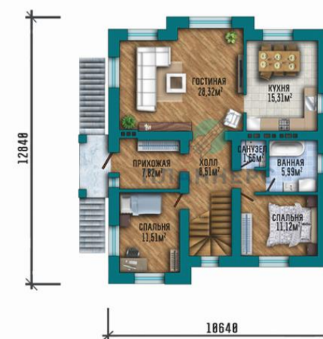
План первого этажа
