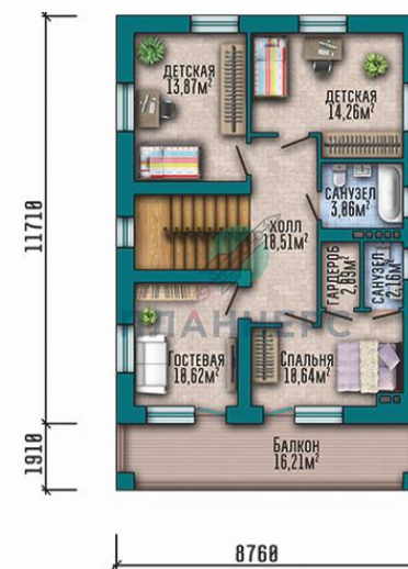
План второго этажа
