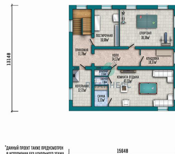
План цокольного этажа
